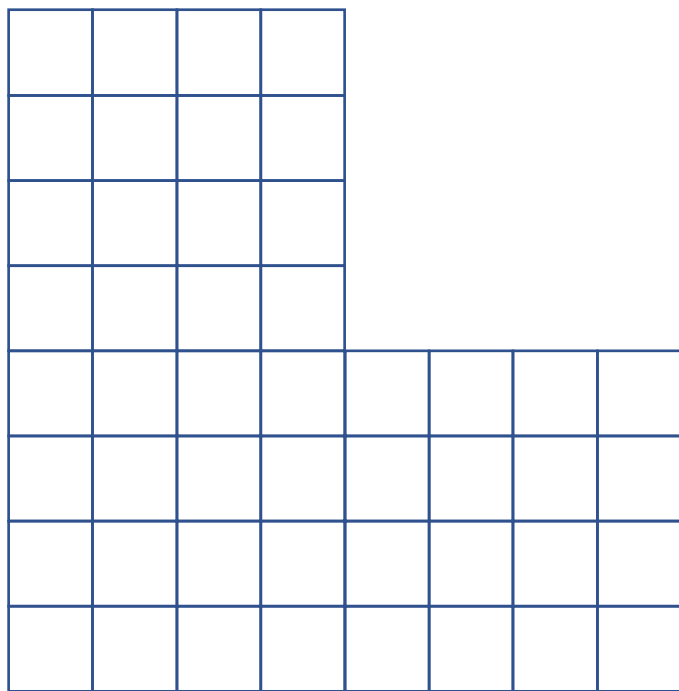
2^k \times 2^k 棋盘
